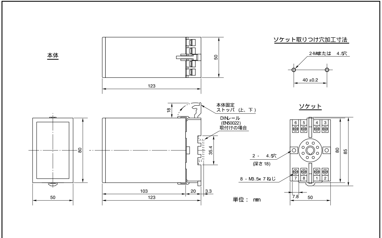
外形寸法図
