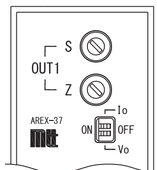
変換器前面
