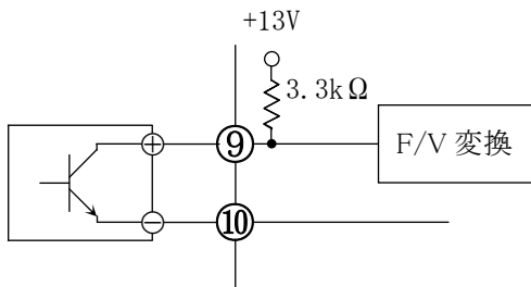
*2線式センサご使用の場合 注:センサの種類により接続の異なる場合があります。
