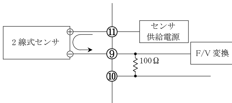
*2線式センサご使用の場合 注:センサの種類により接続の異なる場合があります。
